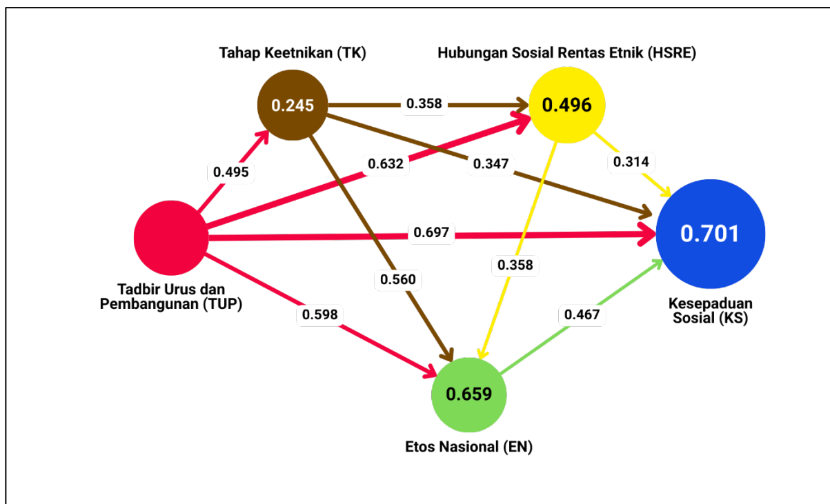
Analisis Berstruktur PLS-SEM Skor Indeks Perpaduan Nasional (IPNas) 2025
