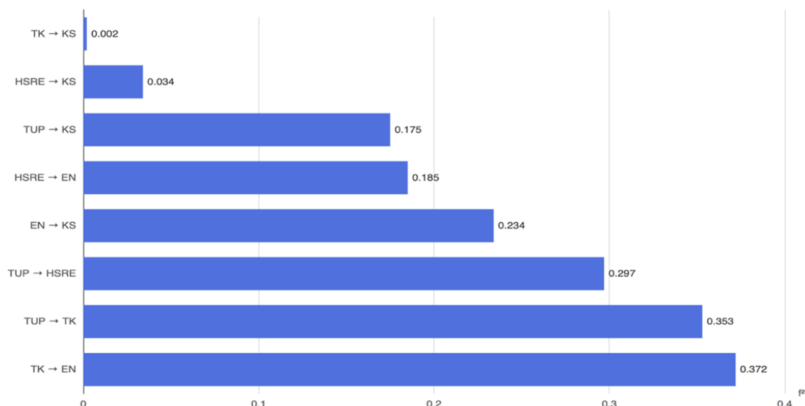
Tahap Kesan Faktor ( f^2 )
